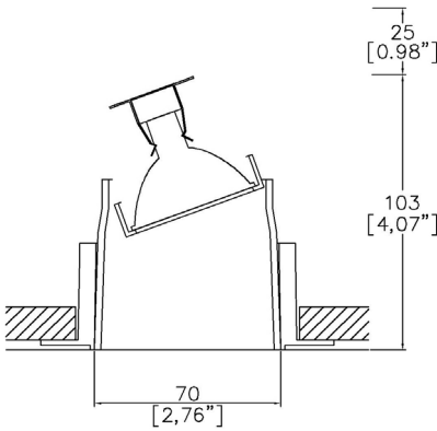
073-MR-TL Cut-out 79mm Ø
